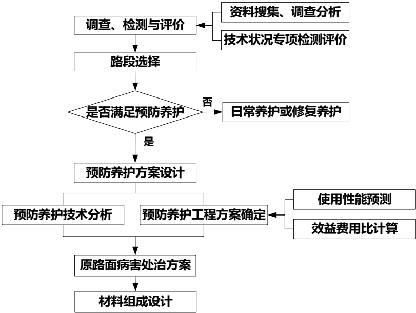
图 1 沥青路面预防养护设计流程
