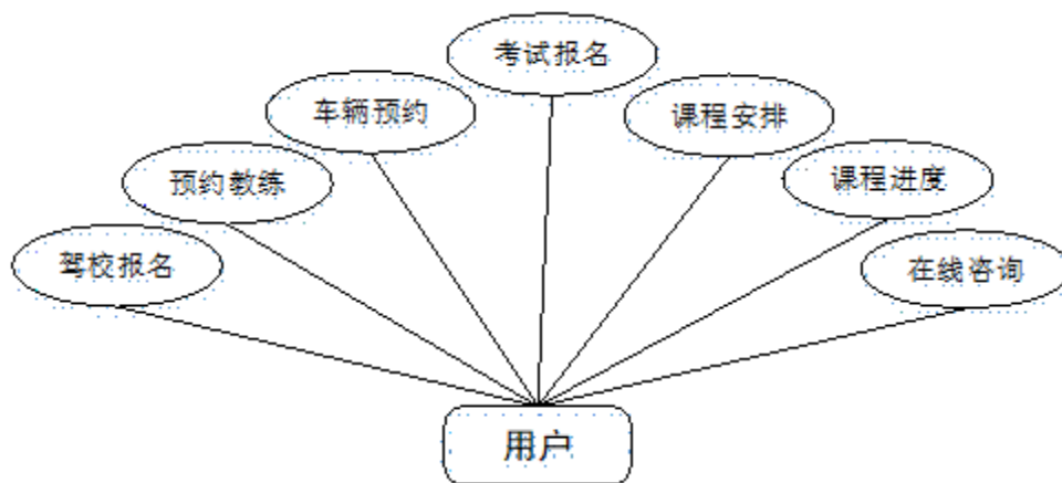
图 3-2 用户用例图
