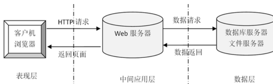
图 2-1 三层结构图
