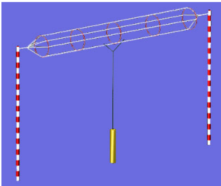
中波天线
