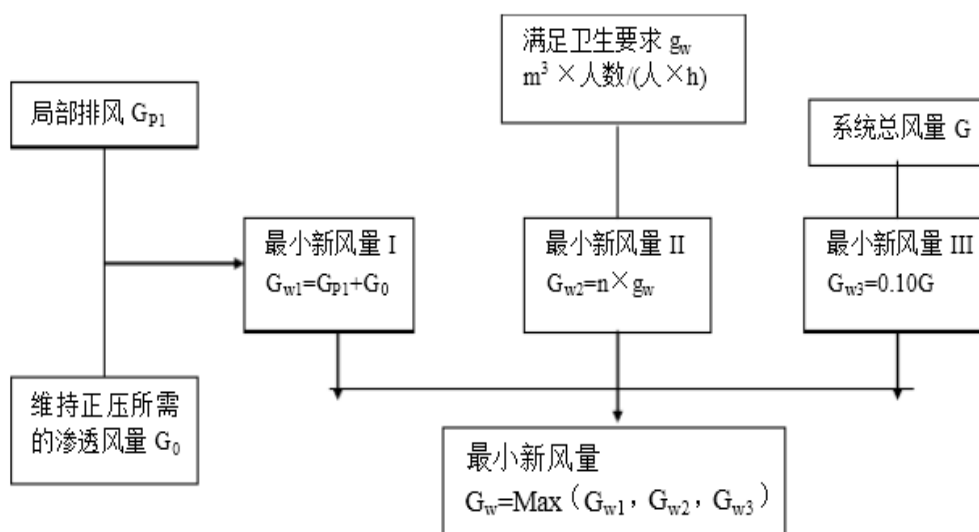
图 4-1 新风量确定示意图框
