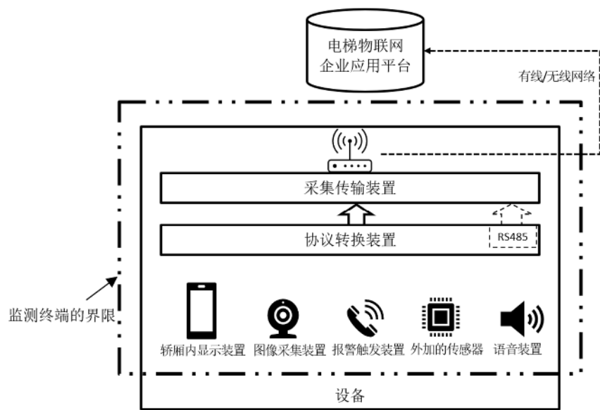
图1 物联网监测终端基本组成示意
