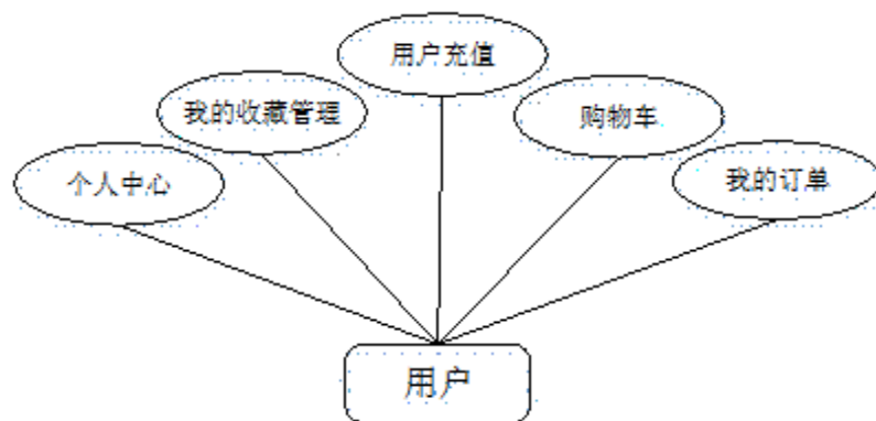
图 3-2 用户用例图
