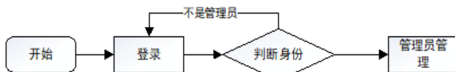
图 3-4 系统流程图
