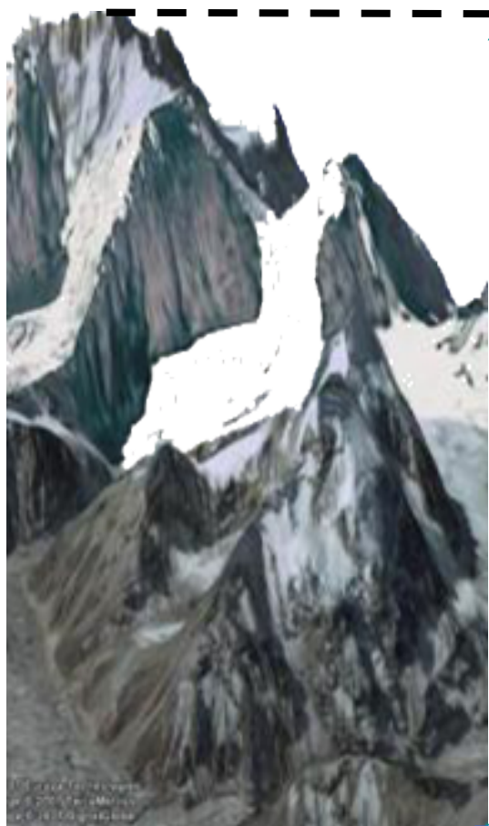
珠穆朗玛峰
