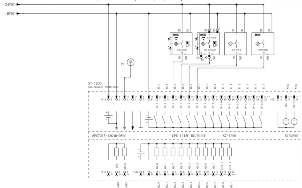
图 1-1-2 传感器安装接线图
