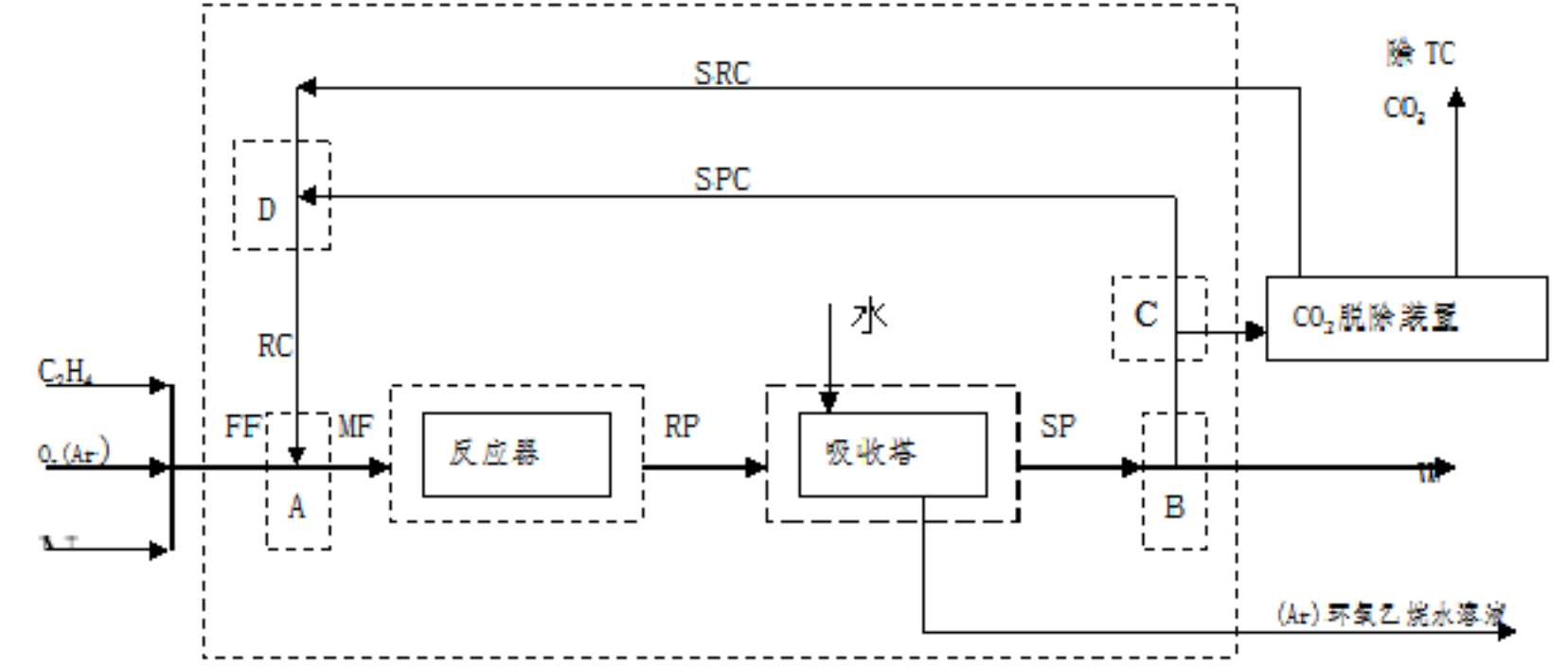
(7) 乙烯催化氧化制取环氧乙烷得物料衡算框图
